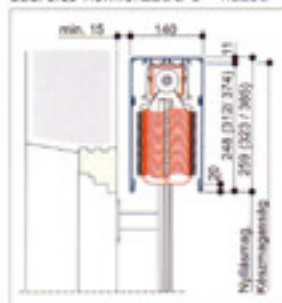
Szerelés homlokzatra íves házba
