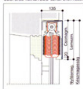
Szerelés falkávéba takarólemezzel
