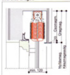
Szerelés üregbe
