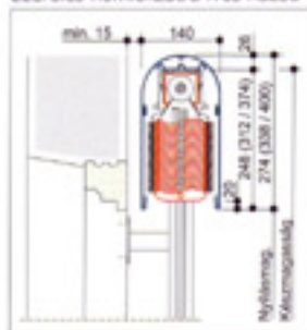
Szerelés üregbe
